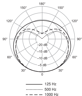
TYPICAL POLAR PATTERNS COURBE DE DIRECTIVITE TYPIQUES - TYPISCHE POLARCHARAKTERISTIK PATRONES DE CAPTACION POLAR TYPICOS - TIPICI DIAGRAMMI POLARI 指向特性
